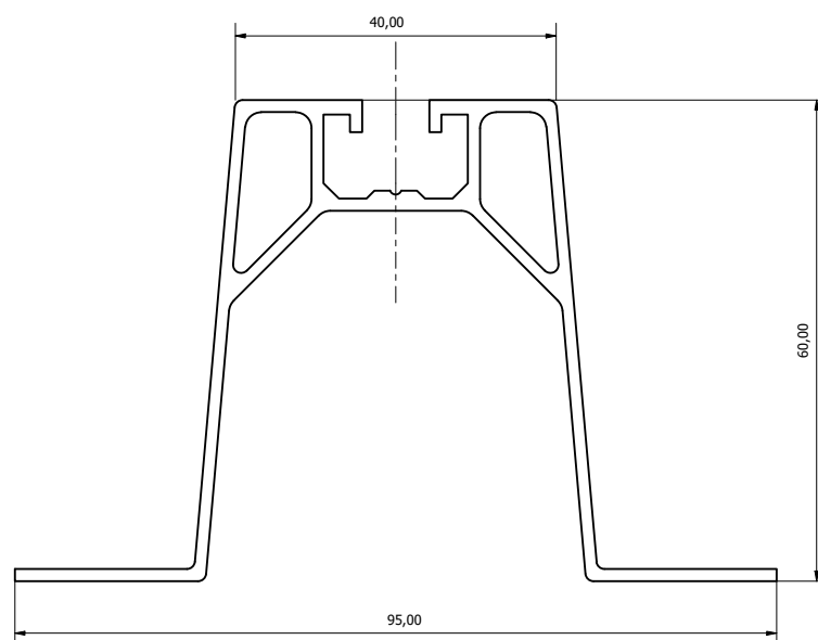
Abb.1 Abmessungen des Elements K-14
